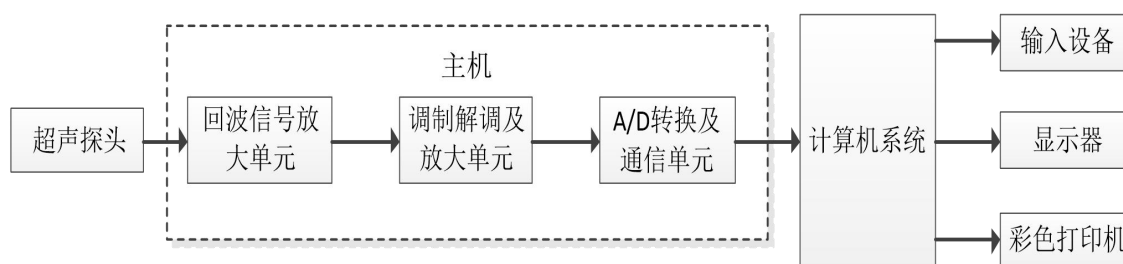
图 1 TCD 仪工作原理结构图
