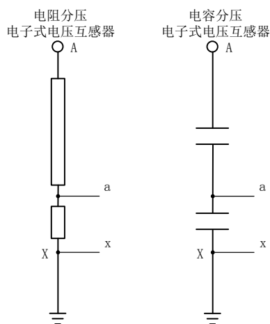
图 1 电子式电压互感器原理图
